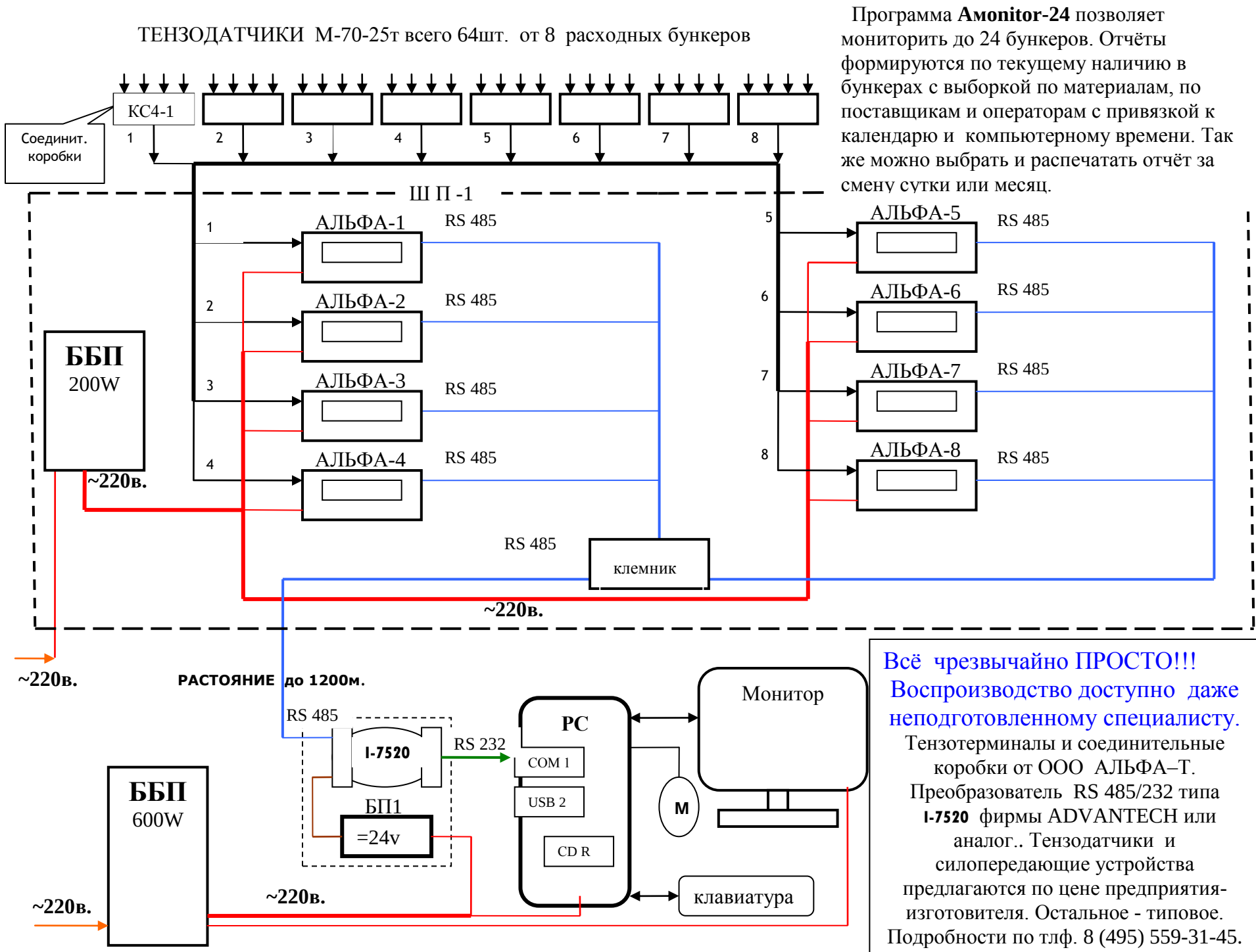
Рис.1 СХЕМА питания и сигналов СИСТЕМЫ СБОРА ИНФОРМАЦИИ для 8-ми 100т. бункеров
